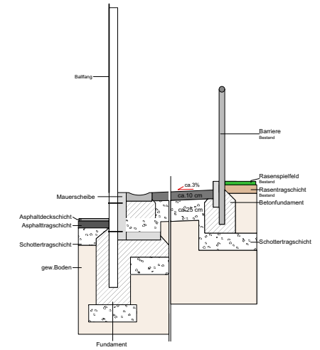
Ansicht Sanierung Weg Ost
