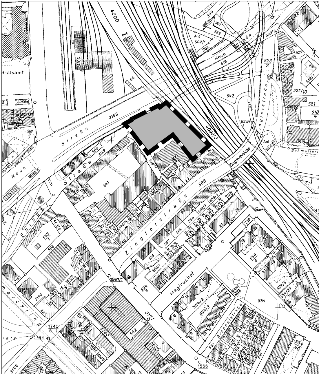
Übersichtsplan M 1 : 2.500
