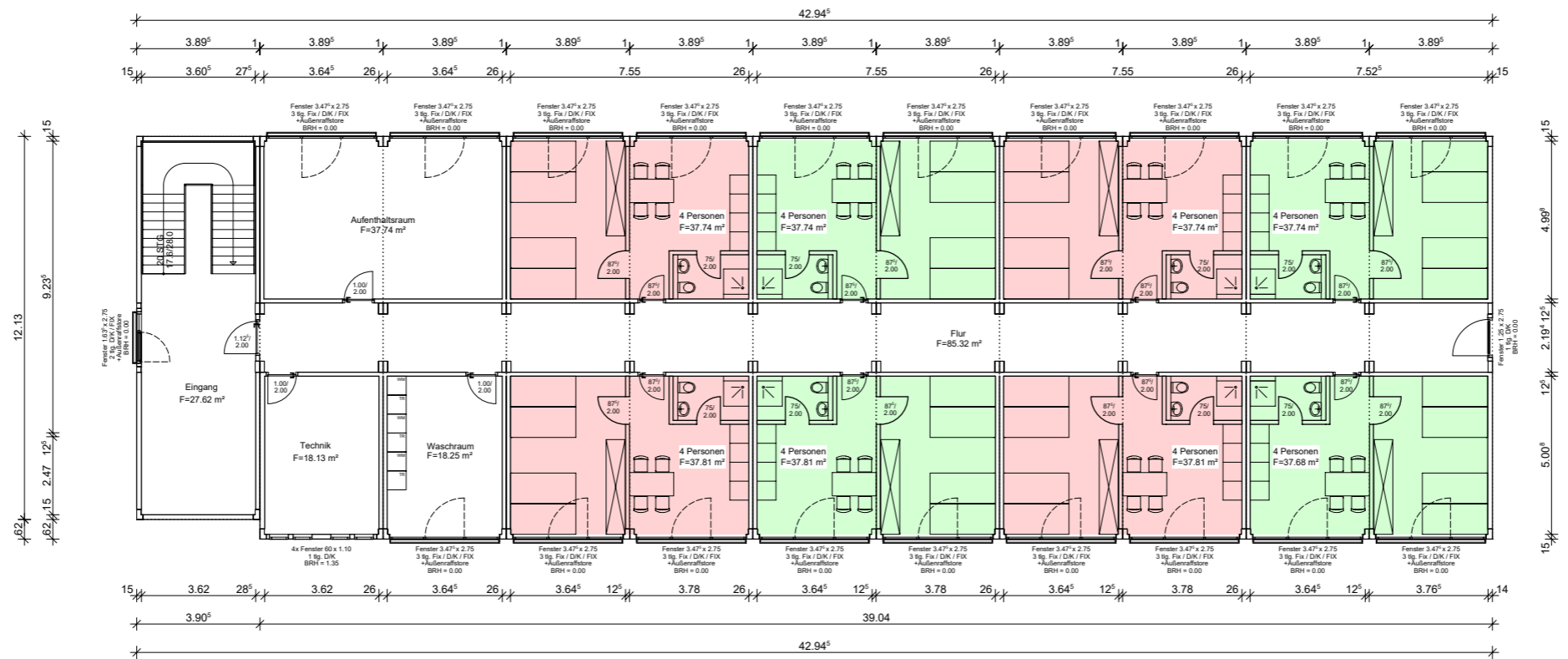
1. Obergeschoss
