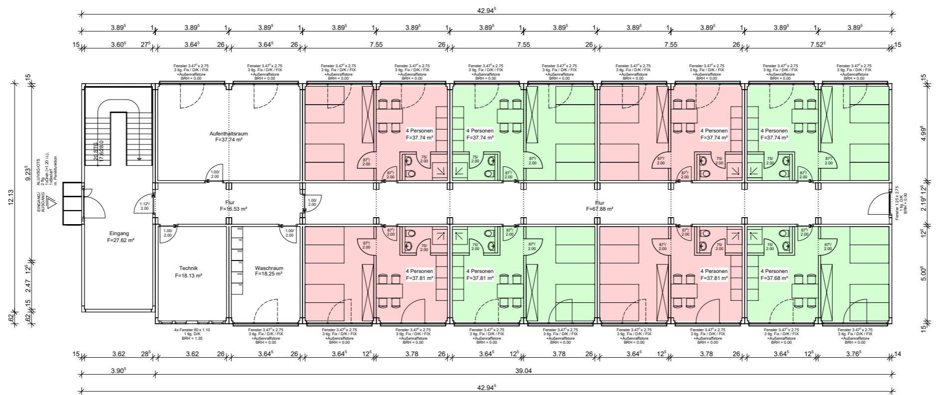
Erdgeschoss
