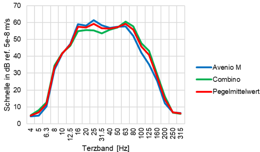
Abbildung 2. Terzbandspektren (Maximalpegel) der Schwingschnelle in dB ref. 5e-8 m/s im Abstand von 8 m zur Gleismitte des Zugtyps Avenio M und Combino sowie Pegelmittelwert der Spektren. Messung im Bereich der Haltestelle Donaustadion.
