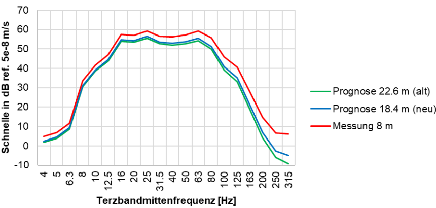
Abbildung 3. Bewertungs-Terzbandspektren (Maximalpegel) der Schwingschnelle in dB ref. 5e-8 m/s im Abstand von 8 m, 18,4 m und 22,6 m zur Gleismitte.
