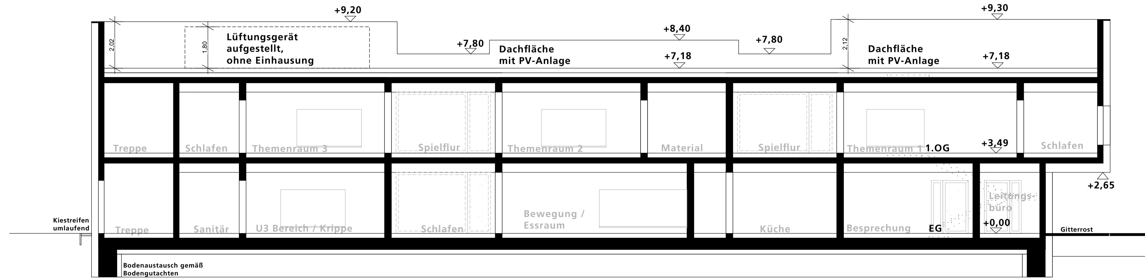
Schnitt BB
