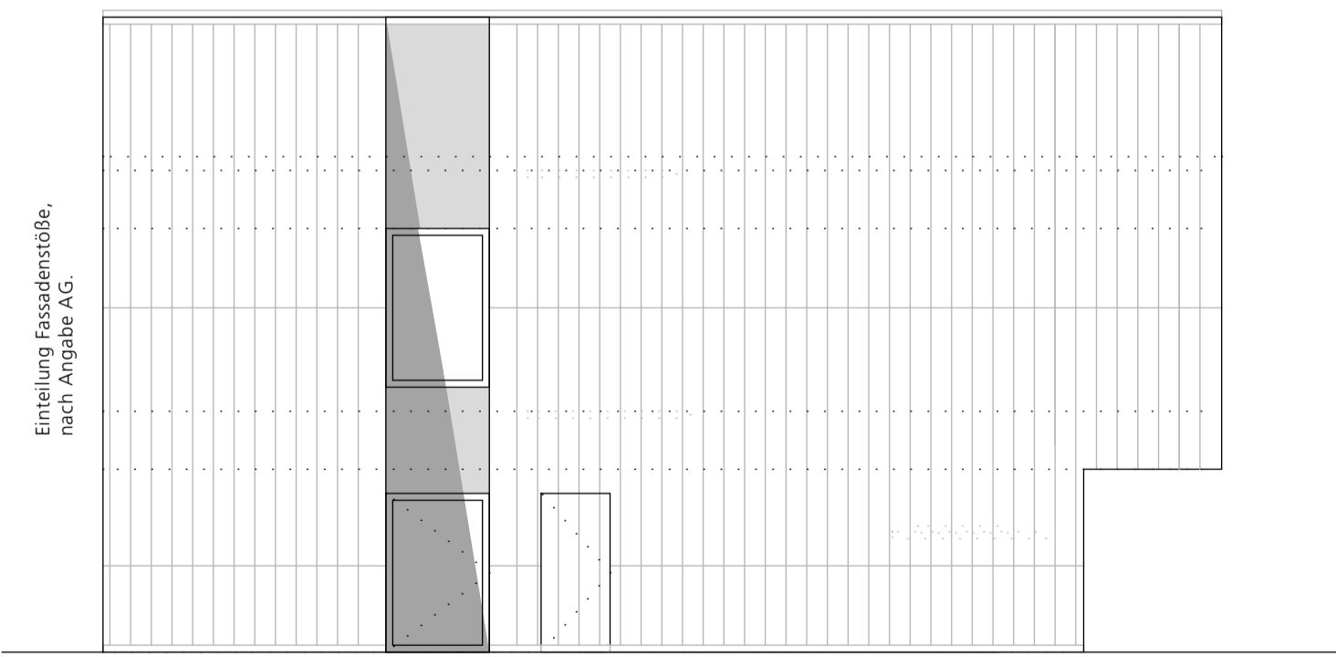
Ansicht Ost
