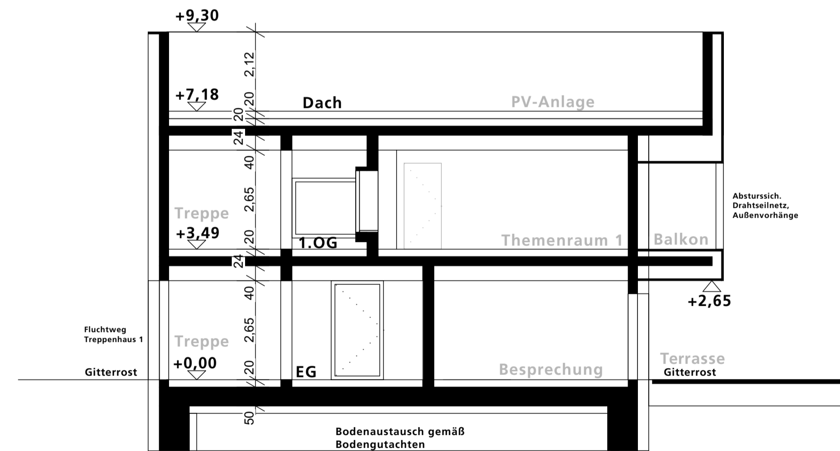
Schnitt AA
