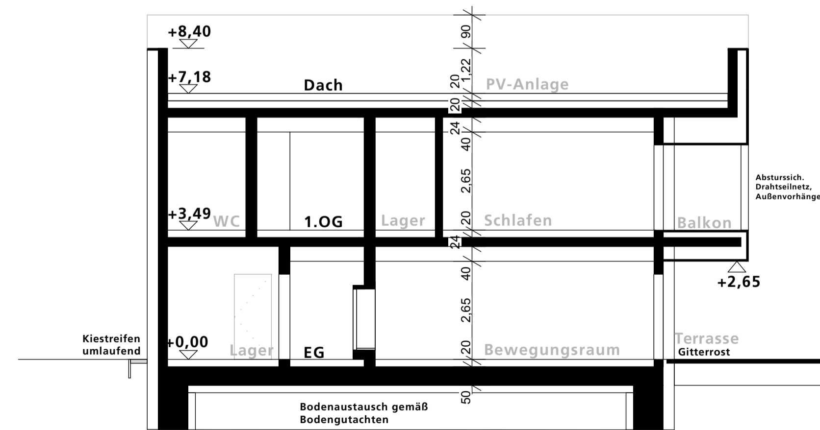
Schnitt CC
