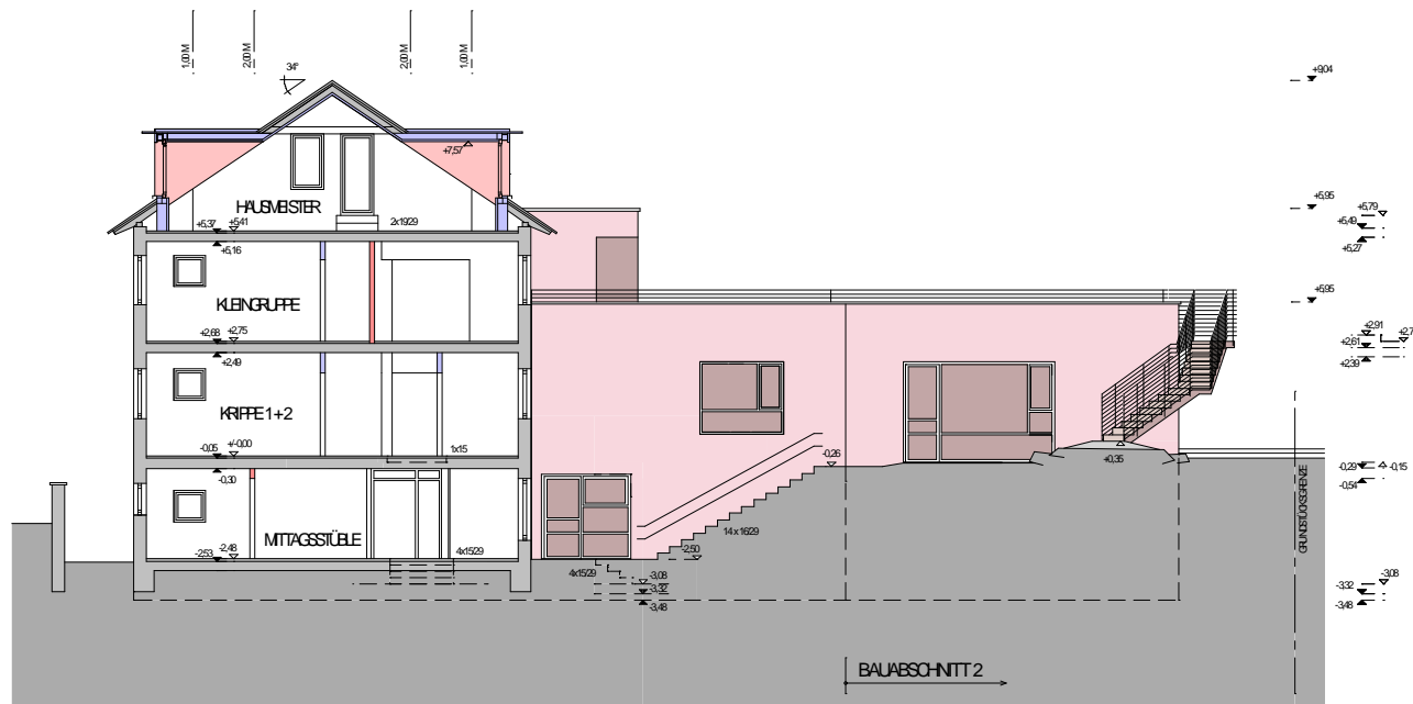
SCHNITT A-A NORDWESTEN
