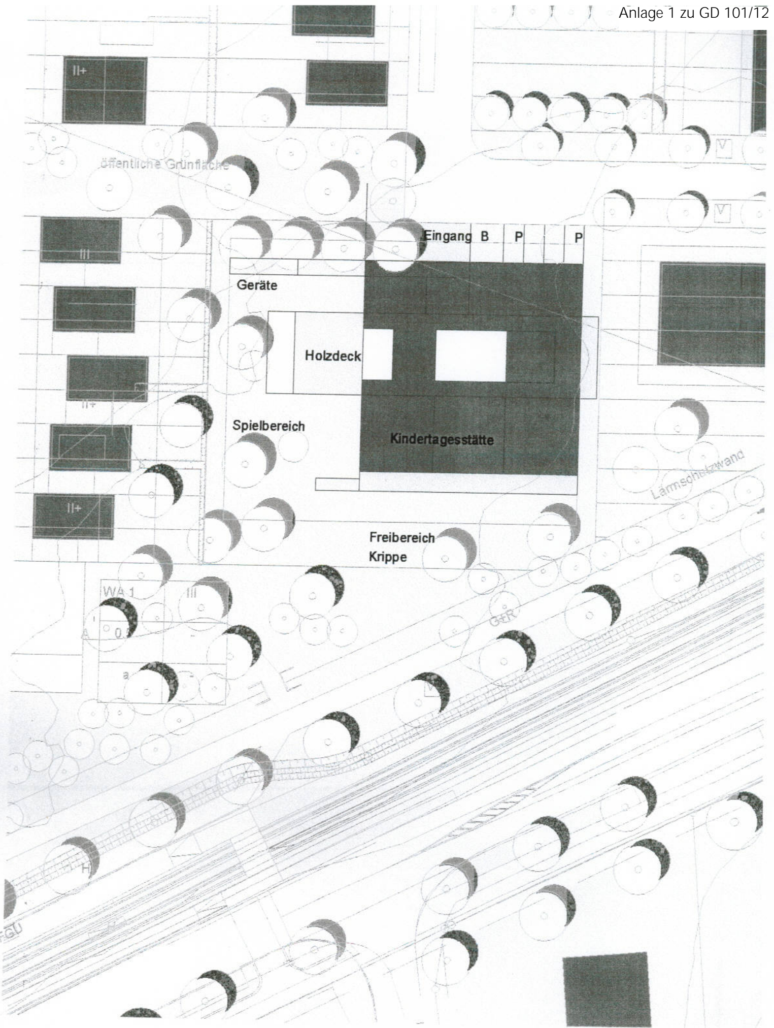
Lageplan M 1:500
