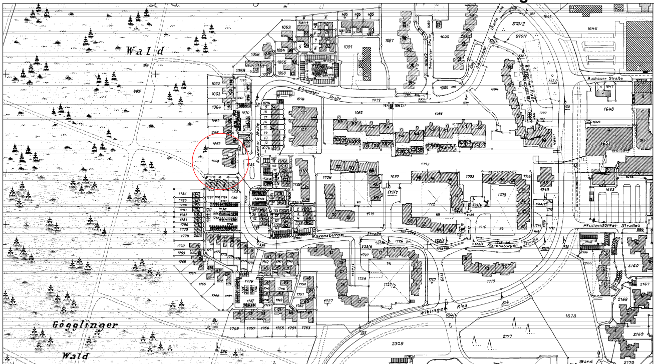
Übersichtsplan Maßstab 1: 5000
