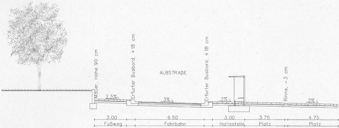
Schnitt B-B'
