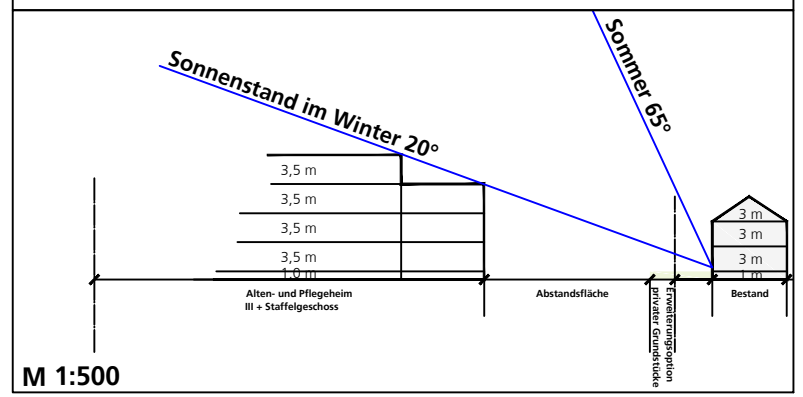
Schemaschnitt A mit Alten- und Pflegeheim
