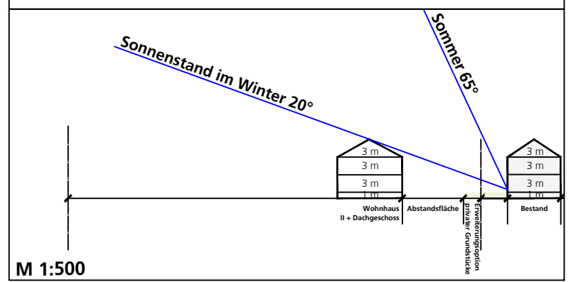
Schemaschnitt A mit Wohnbebauung (zum Vergleich)
