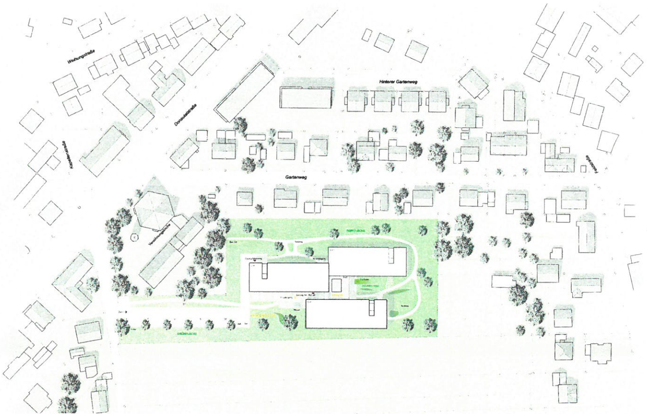
LAGEPLAN 1:500
