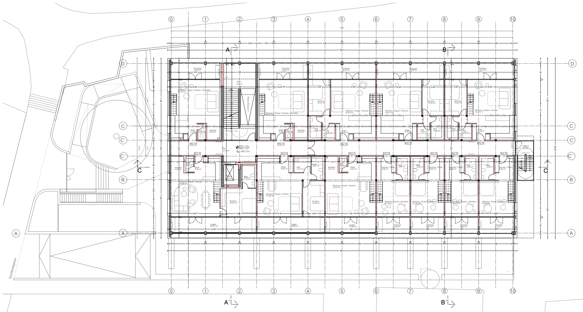
Grundriss 1. OG
