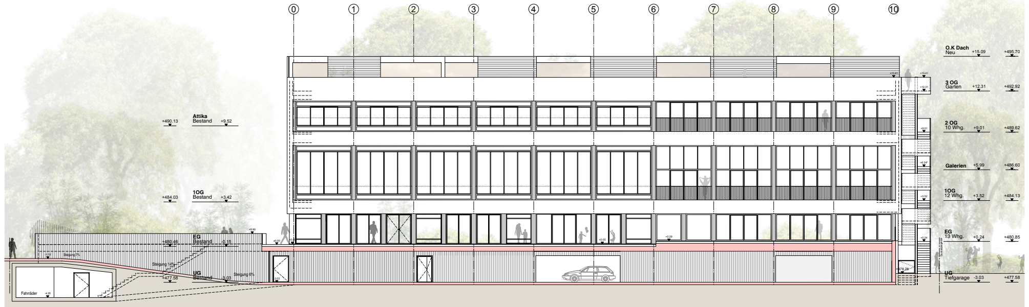
Ansicht Süd
