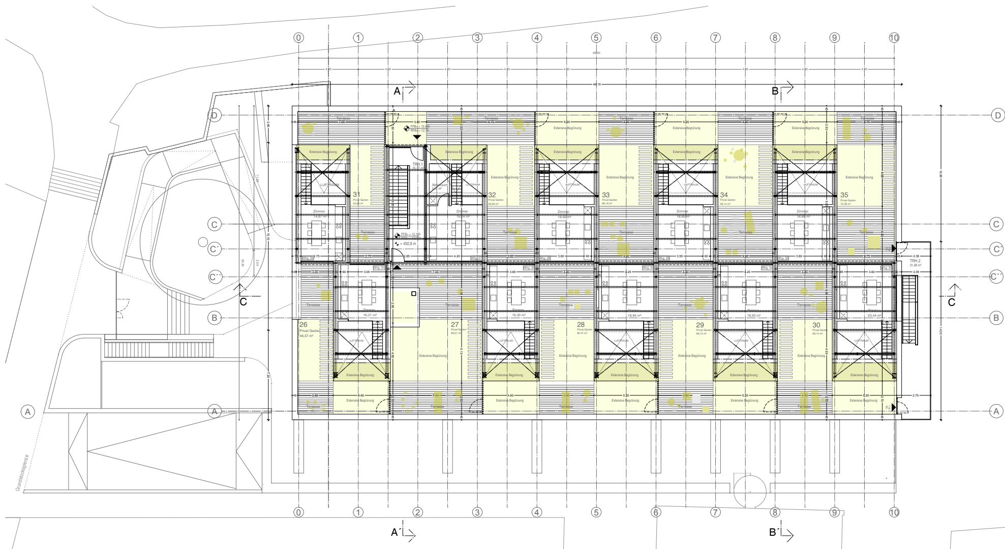
Grundriss DG
