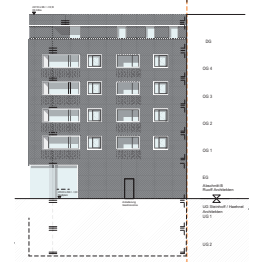
Strassenansicht Abschnitt B Ost
