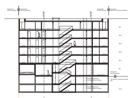
Schnitt Abschnitt B
