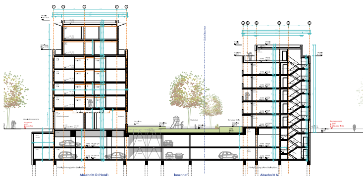
Schnitt B-B - Hotel + Abschnitt A
