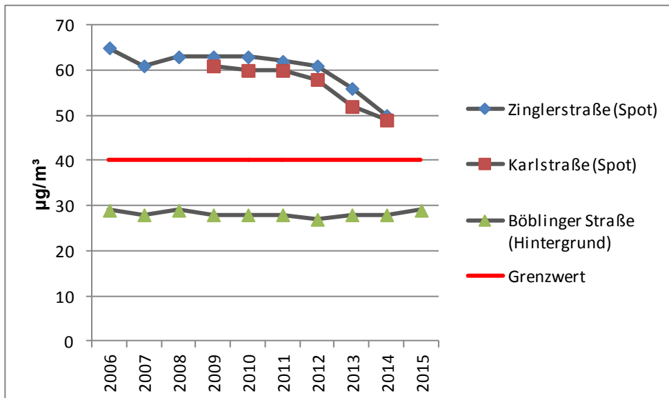
Grafik 2: \text{NO}_2 -Jahresmittelwerte für Ulm an den verschiedenen Messstationen in Ulm
