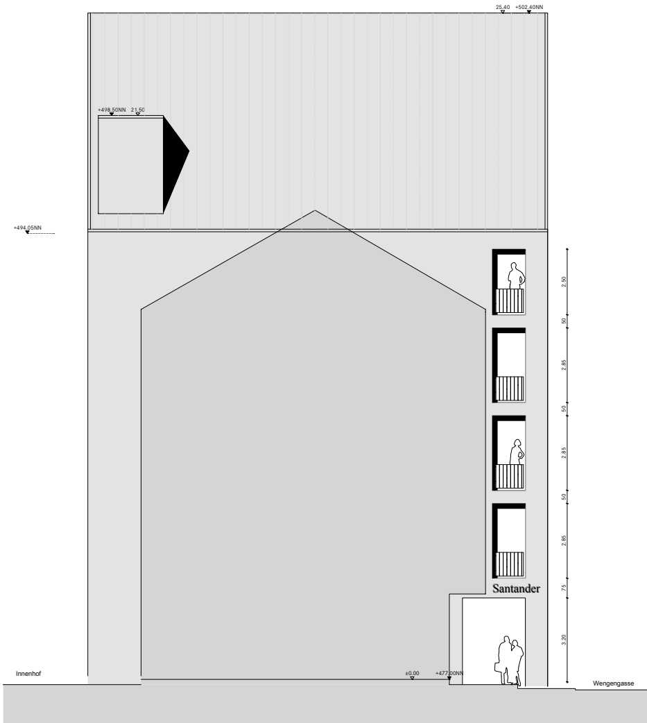
ANSICHT SÜDSEITE M: 1_200
