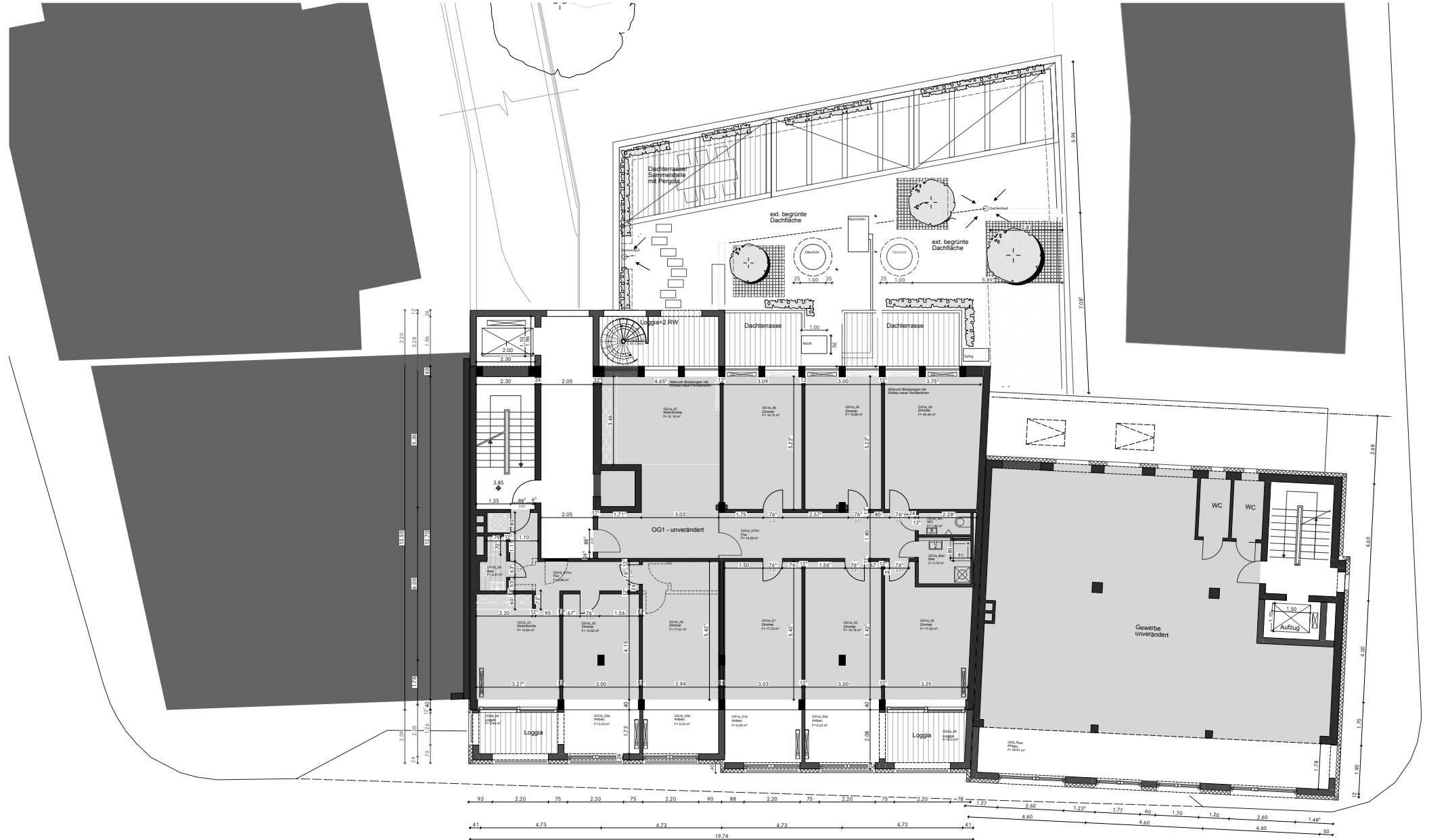
1.OBERGESCHOSS M: 1_200
