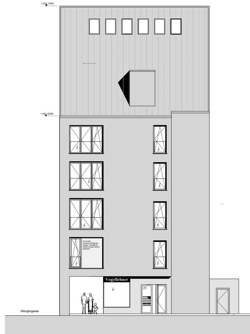
ANSICHT NORDSEITE M: 1_200
