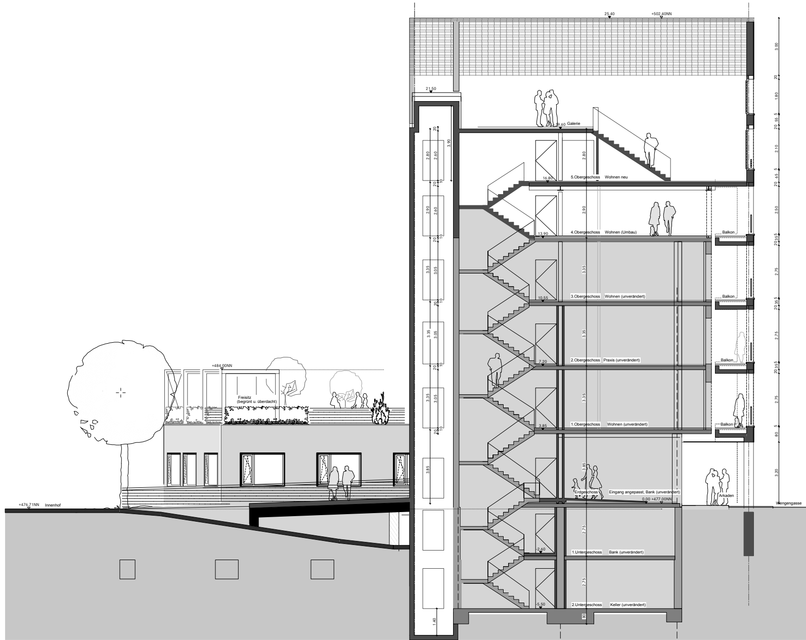
QUERSCHNITT M: 1_200
