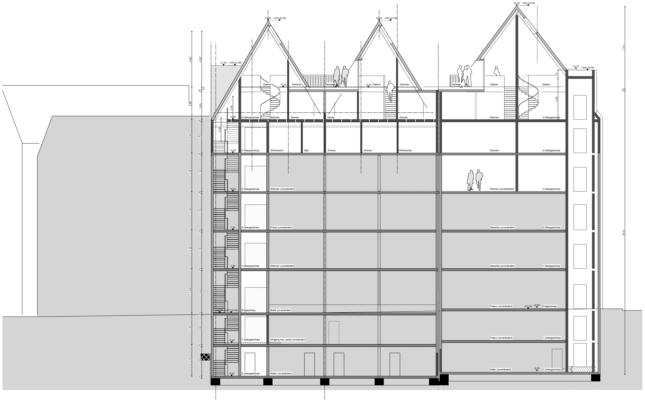
LÄNGSSCHNITT M: 1_200
