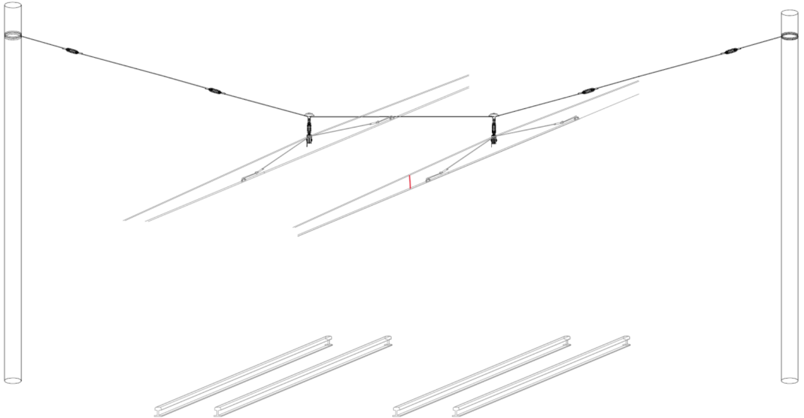
Einfachfahrleitung mit Verstärkerseil
