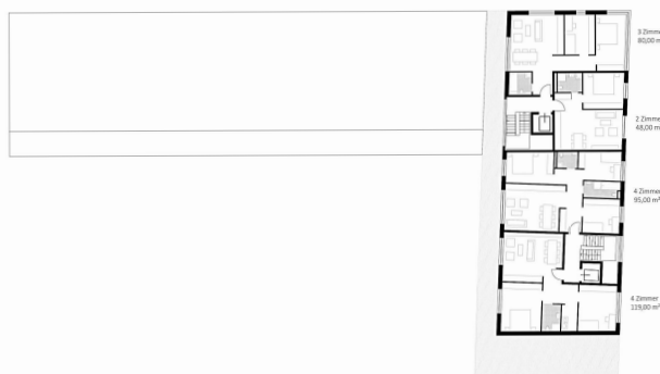
Grundriss Dachgeschoss M 1:200
