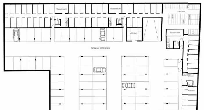
Grundriss Untergeschoss M 1:200
