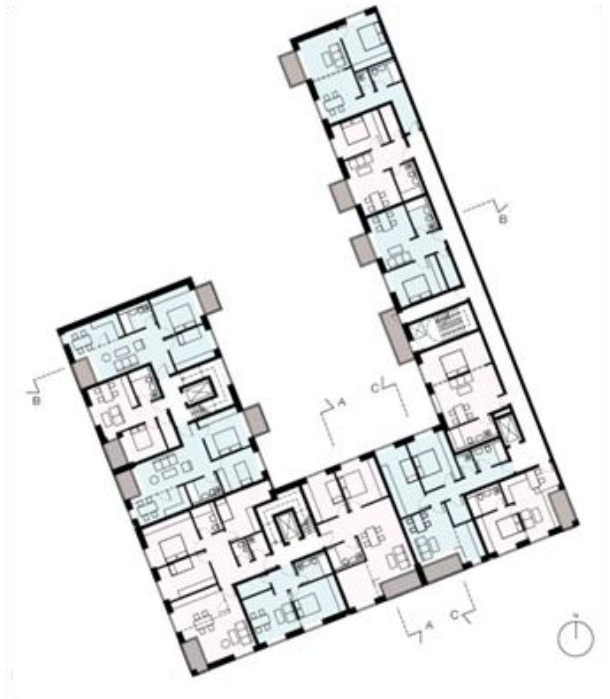
Grundriss Regelgeschoss
