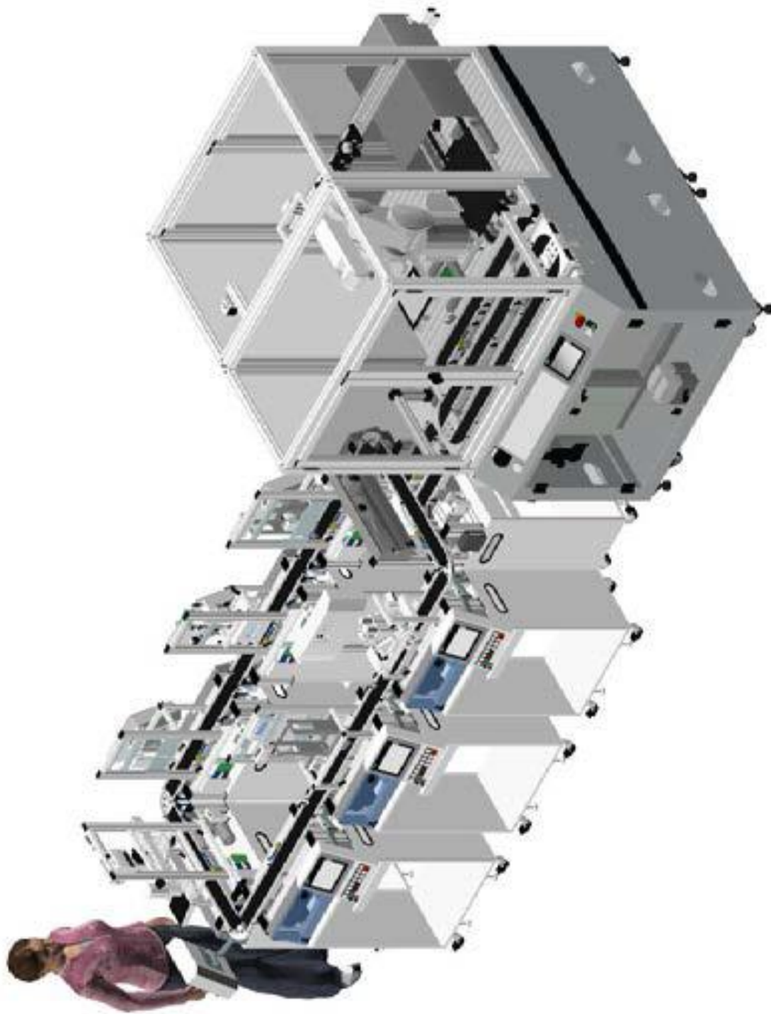
Lernfabrik 4.0 an der Robert-Bosch-Schule Ulm: Gesamtanlage mit Roboterstation
