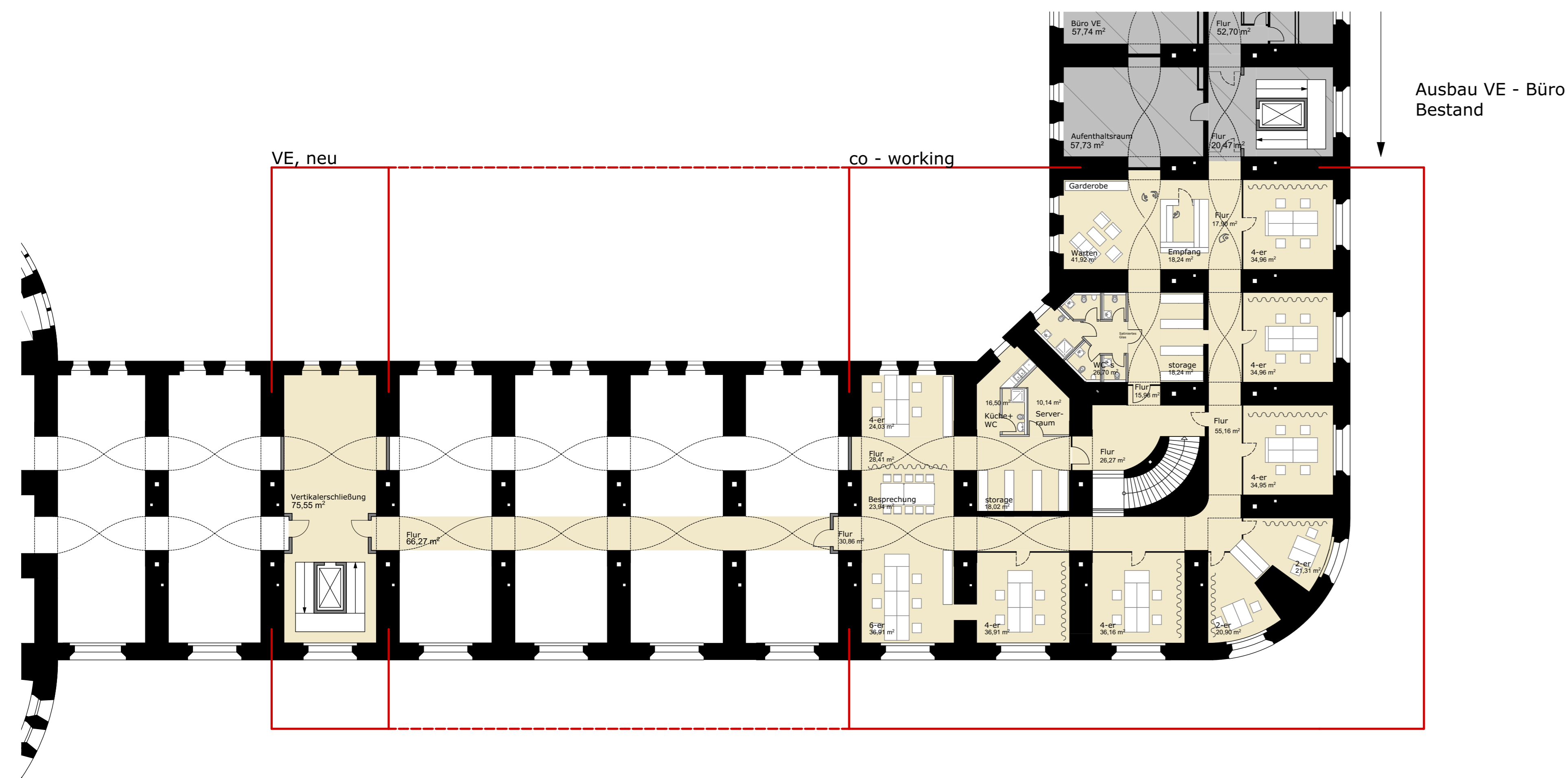
Grundrissauszug 1.OG , M. 1:200
