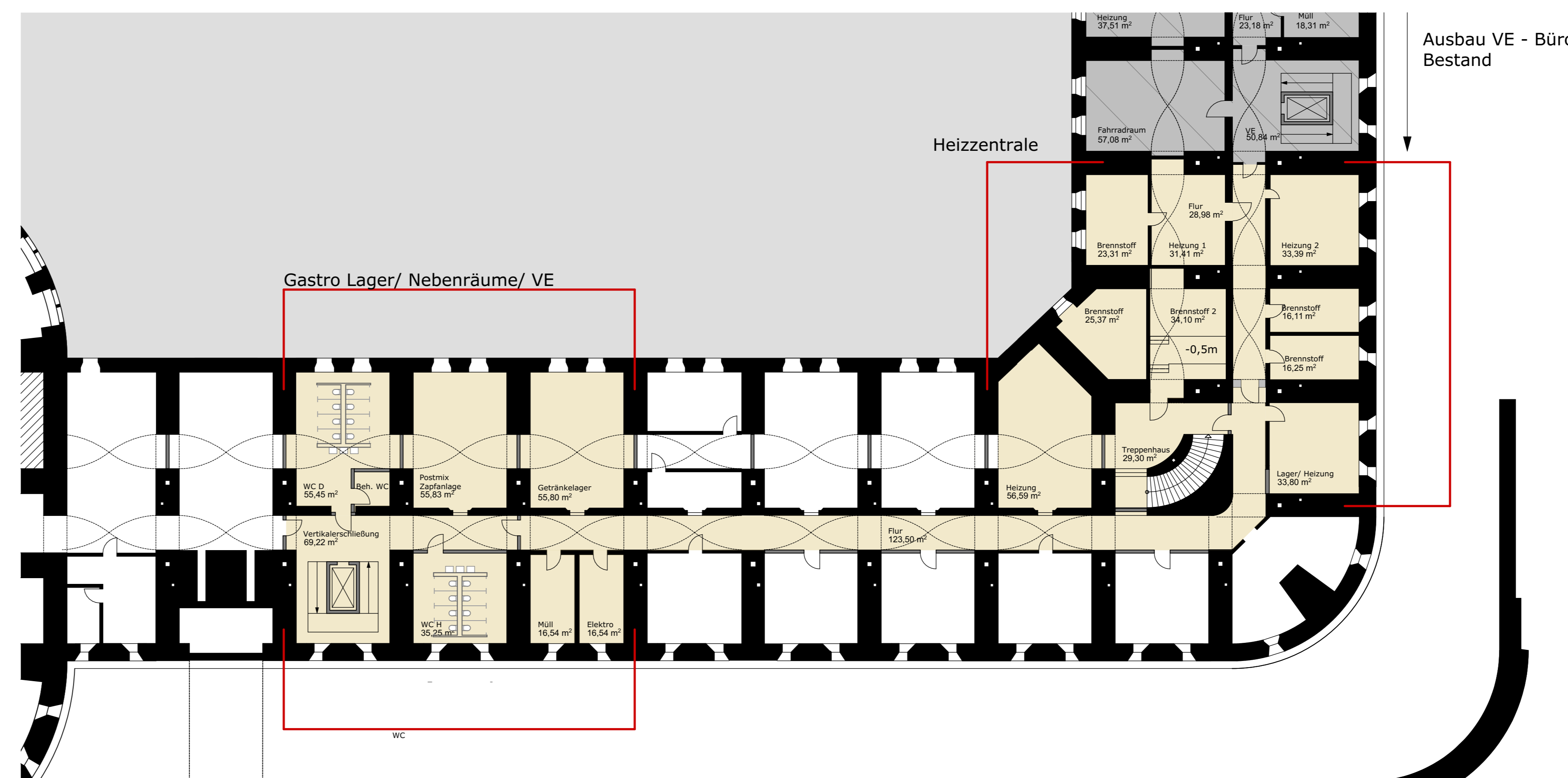
Grundrissauszug Lager/ Heizung UG , M. 1:200
