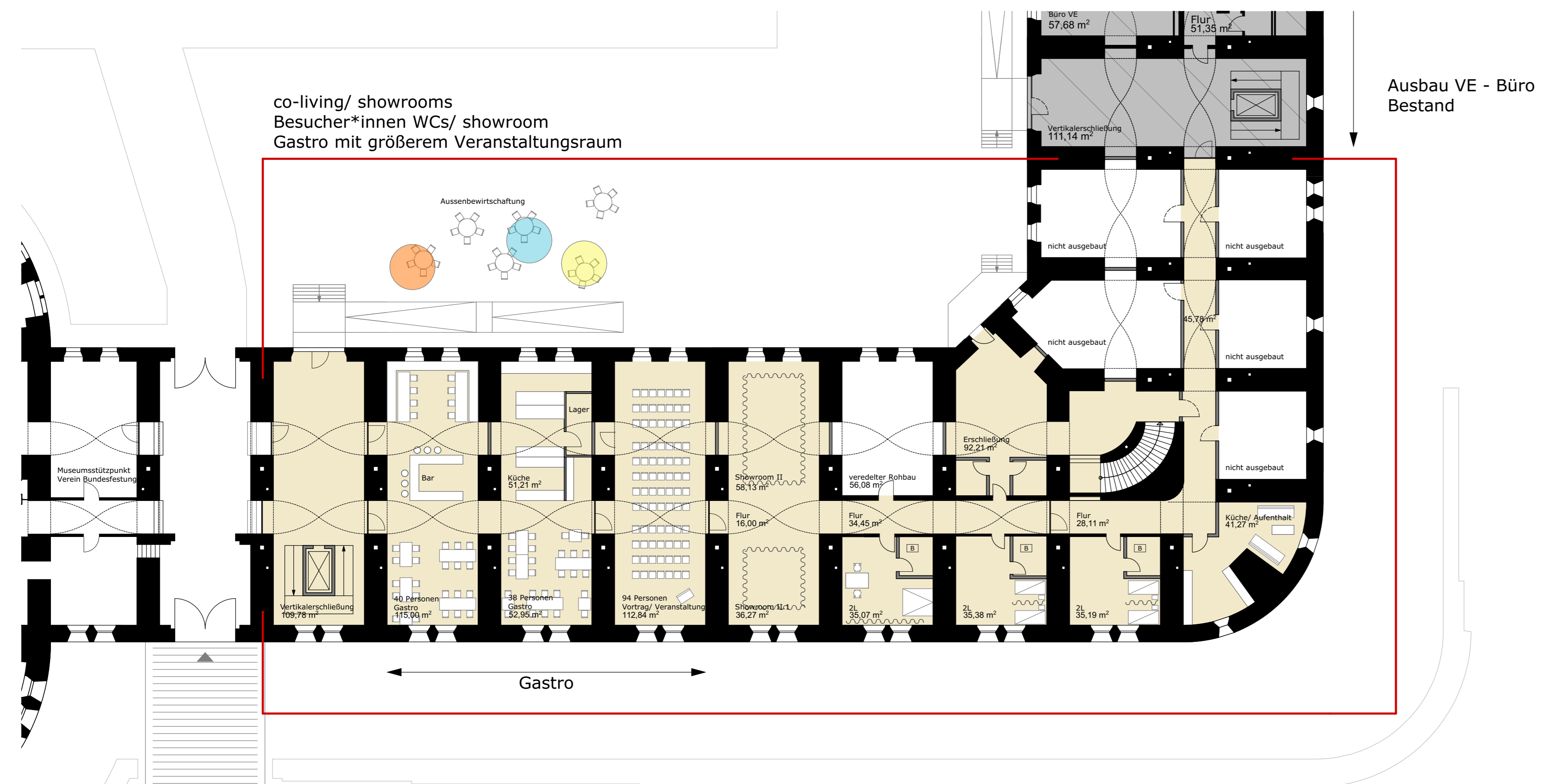
Grundrissauszug EG , M. 1:200
