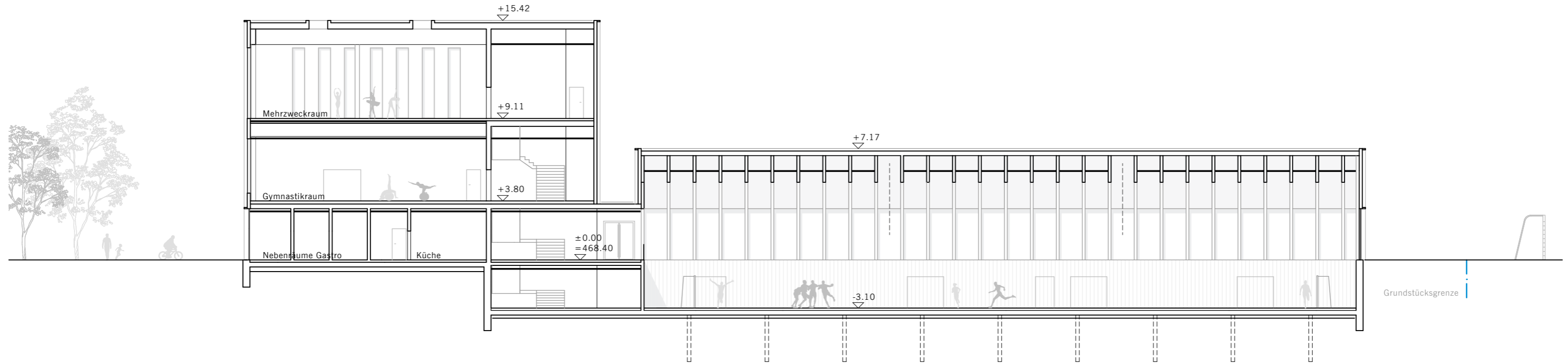
Schnitt 11
