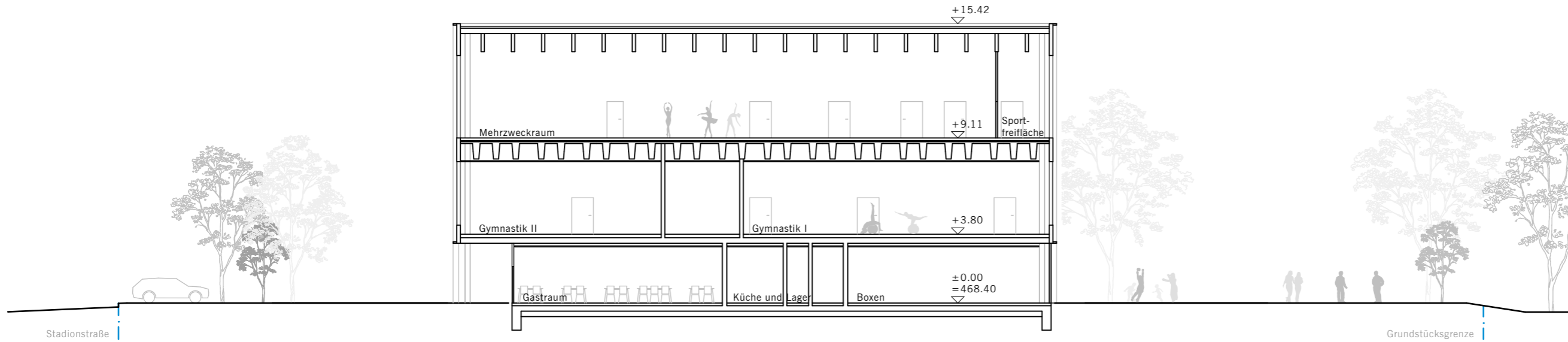
Schnitt AA
