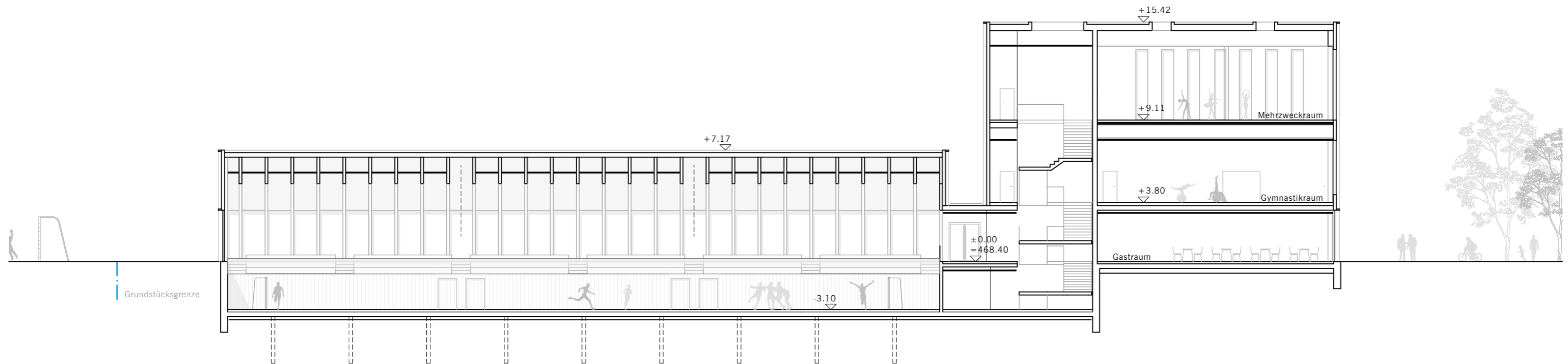
Schnitt 22
